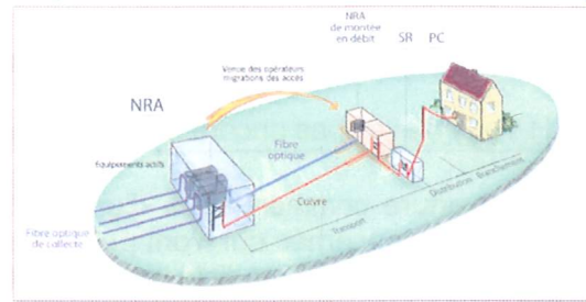
Figure 2 Reaménagement de la boucle locale pour la montée en débit sur fil de cuivre
